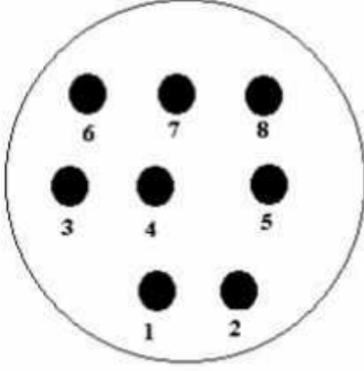
8 PIN ERKEK KONNEKTOR DIŞ GÖRÜNÜŞ
